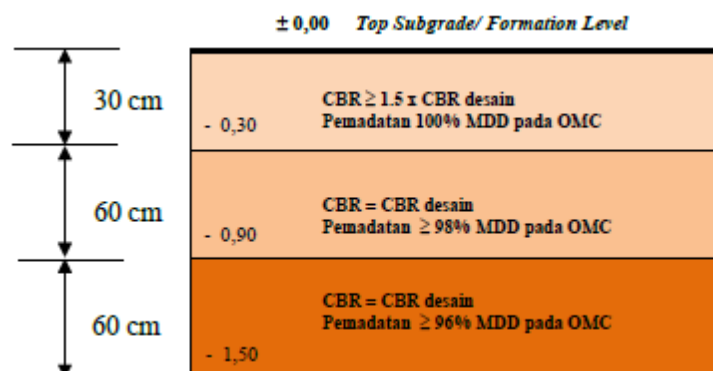
Gambar 3.6.2 Kriteria Pemadatan Subgrade untuk Code Letter D, E dan F
