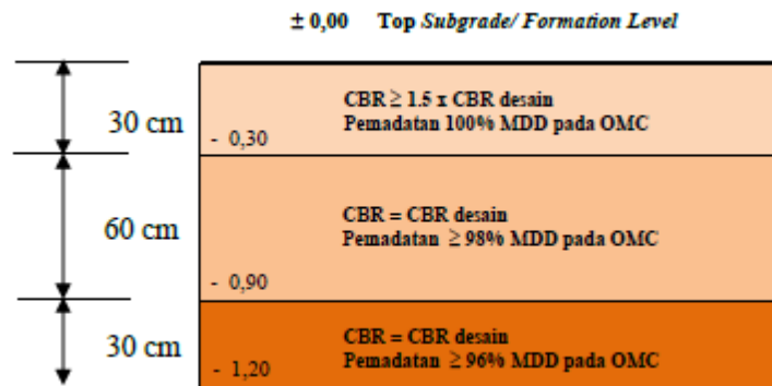
Gambar 3.6.1 Kriteria Pemadatan Subgrade untuk Code Letter C
